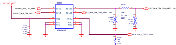
N79 DPDT2 主板
